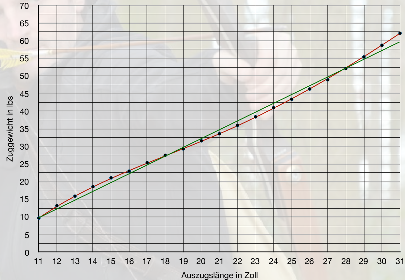
Auszugsdiagramm
